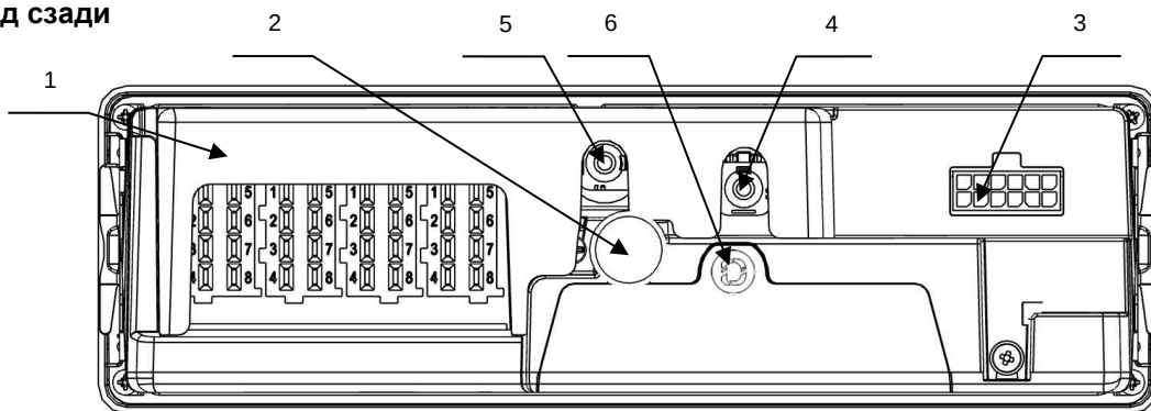
Рисунок 4. Вид сзади
