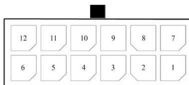
Рисунок 5. Нумерация контактов разъема Molex 43045–1200
