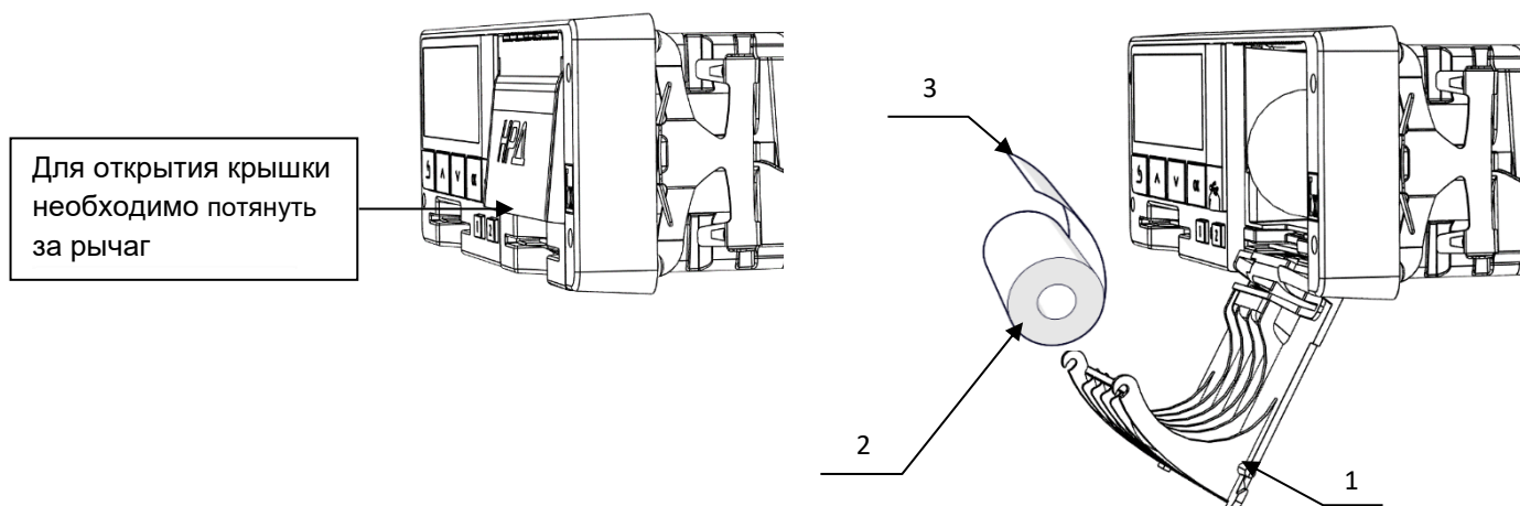
Рисунок 7. Установка бумаги
