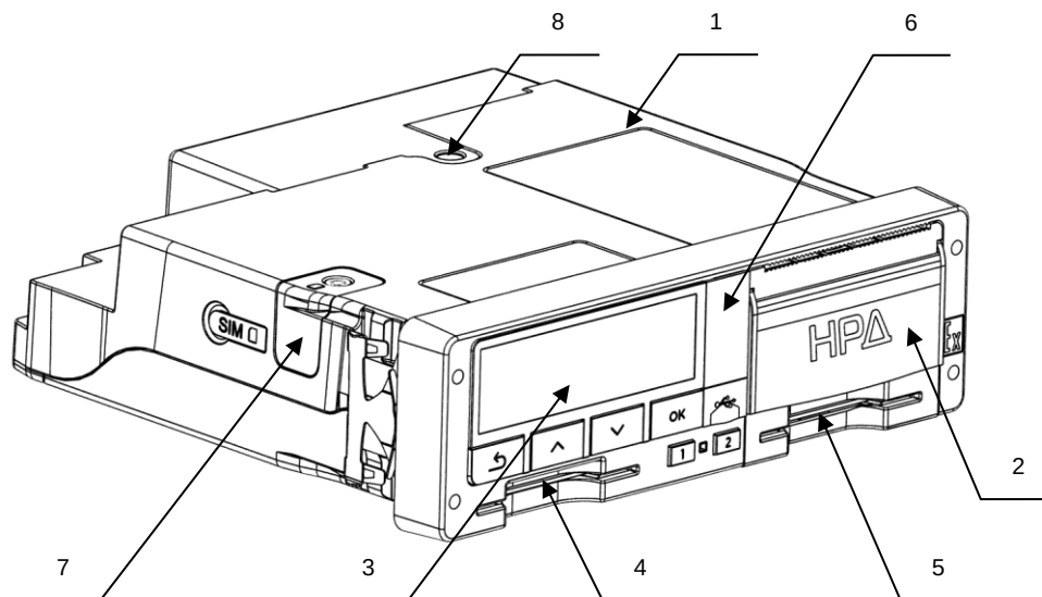
Рисунок 2. Внешний вид тахографа
