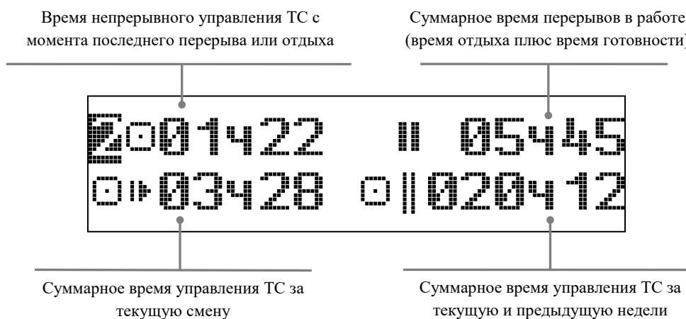
Рисунок 12. Экран «Водитель 2»
