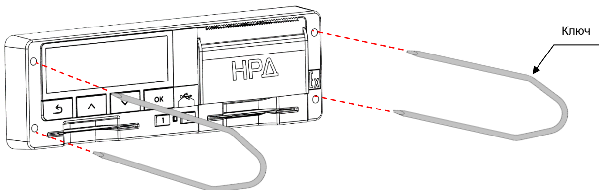
Рисунок 1. Извлечение тахографа
