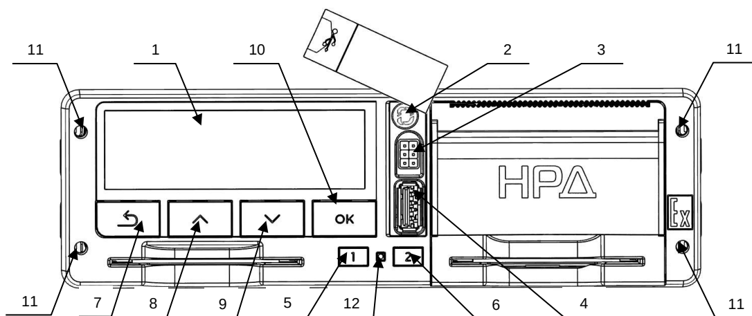
Рисунок 3. Вид спереди
