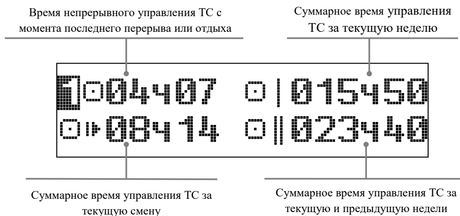
Рисунок 11. Экран «Водитель 1»
