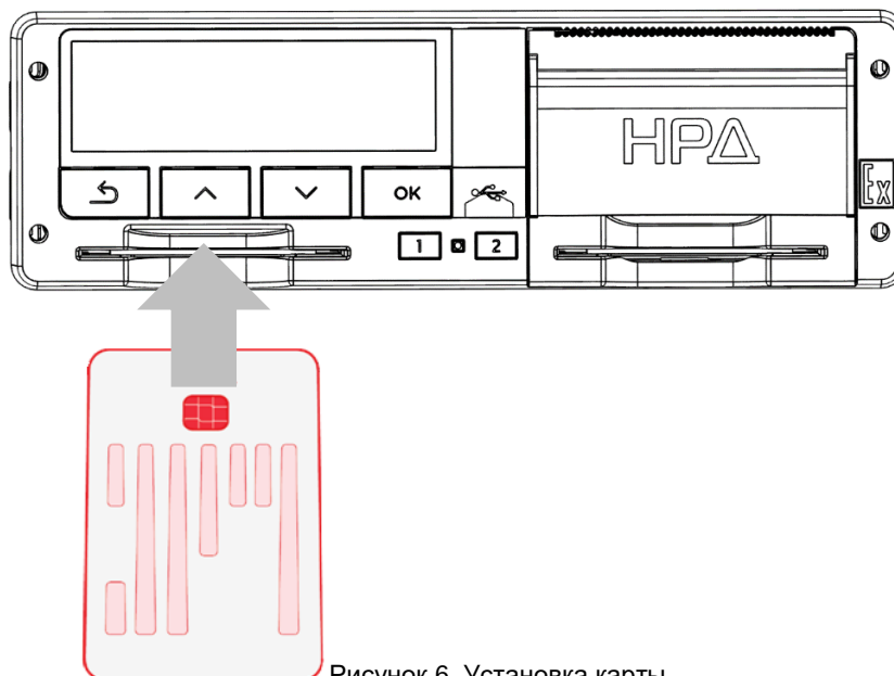
Рисунок 6. Установка карты
