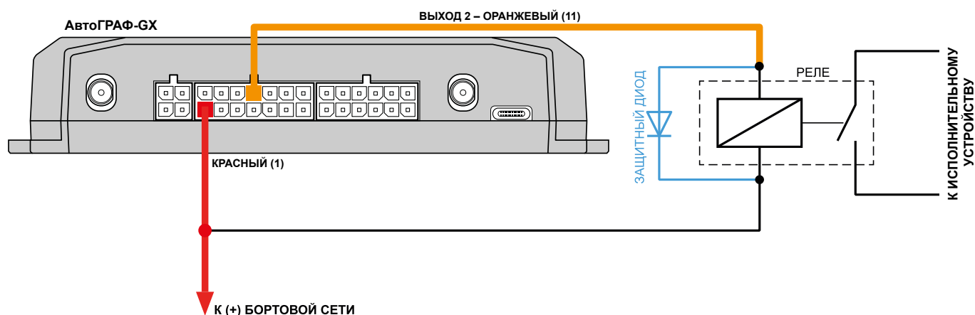
Рис.15. Подключение выхода.
