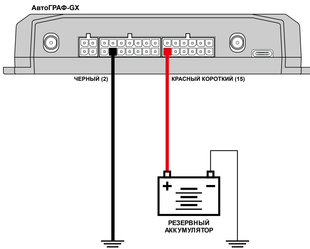
Рис.8. Установка резервного аккумулятора.
